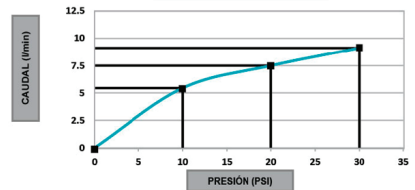
GRÁFICO DE PRESIÓN VS CAUDAL
